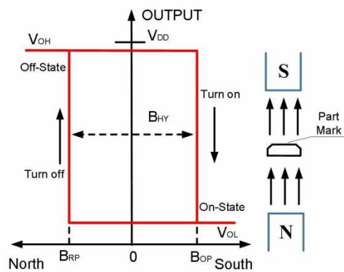
TO-92S封装输出曲线
