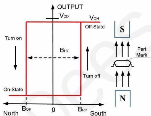
SOT-23-3L封装输出曲线
